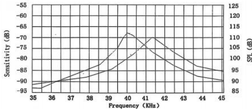
灵敏度/声压级 (10Vrms、30cm)
